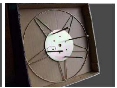
2,500m巻きPPバンドの場合は外側の穴に、長い方の芯を4本セットして下さい
